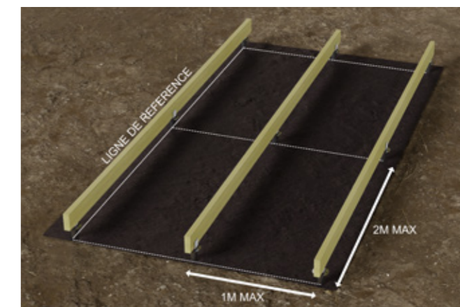
Exemple pour structure croisée en pin avec solives 45x145mm et lambourdes 45x70 mm
