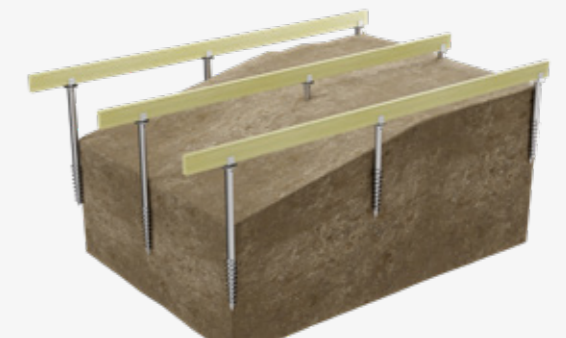
Etape 2 Pose des solives
